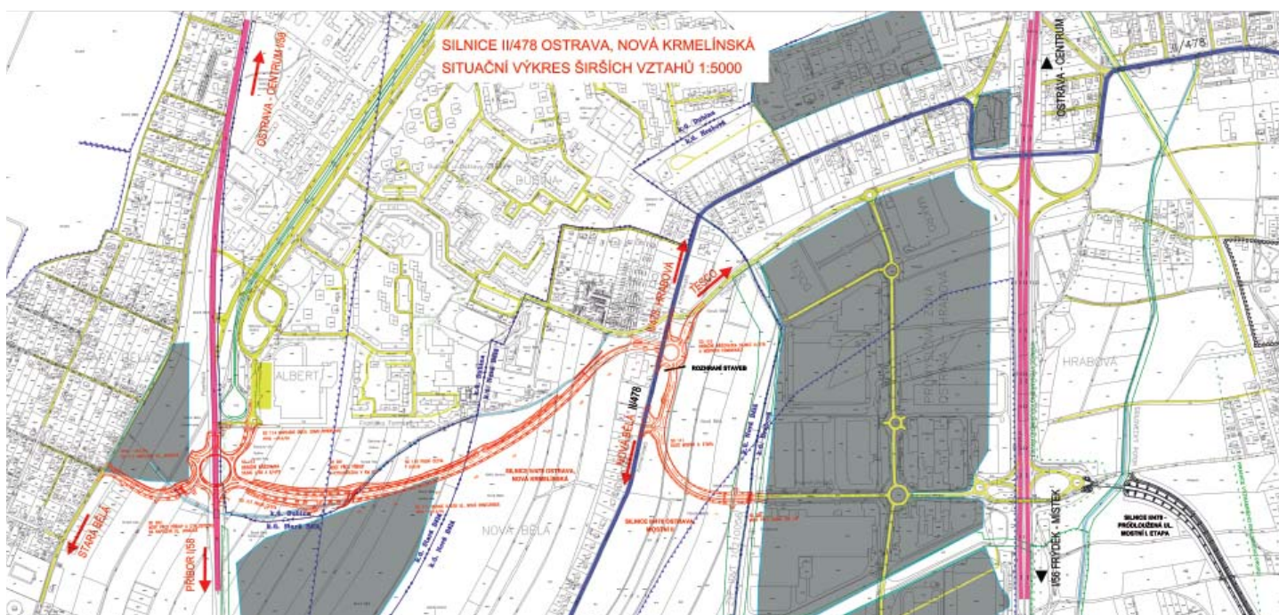
Výkres, na kterém je vidět plánované propojení Nové Krmelínské s Mostní II.
